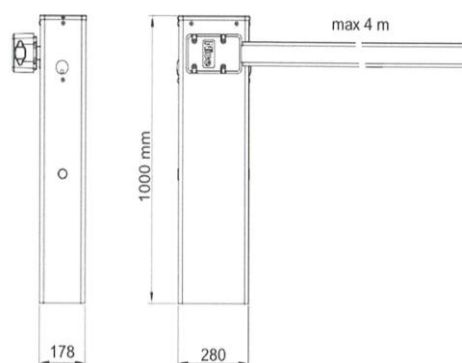
Габариты
